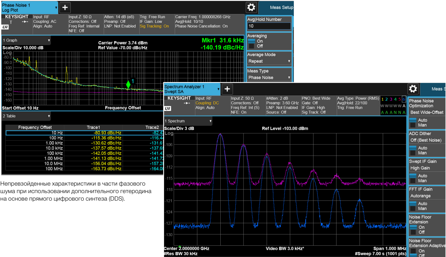
Точное измерение сигналов низкого уровня путем снижения зашумленности результатов измерений до 10 дБ благодаря функции понижения уровня собственных шумов (NFE).
